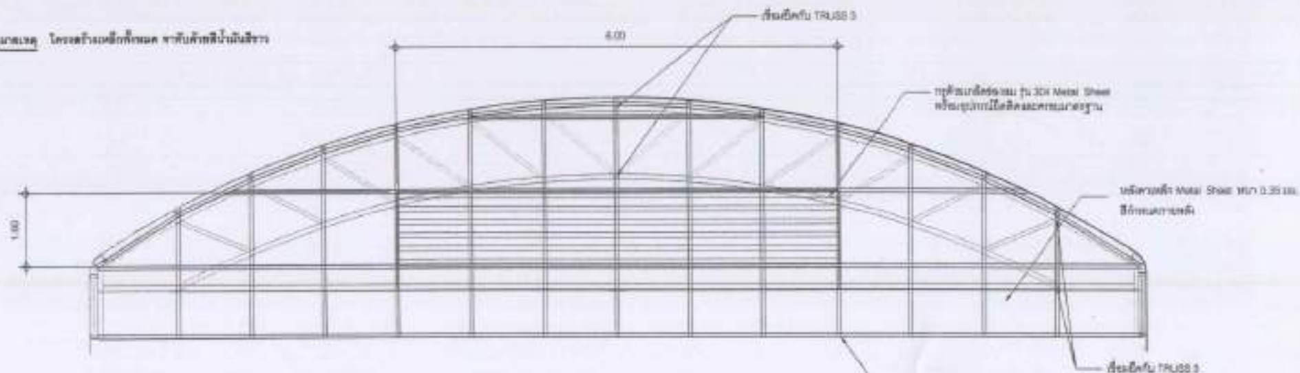
แบบขยาย TRUSS 4
