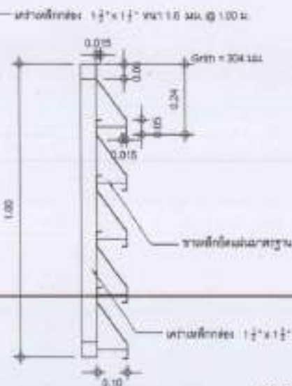
แบบขยายเหล็กโครงสร้าง
