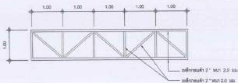
แบบขยาย TRUSS 3
