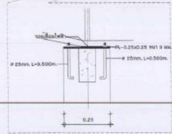
แบบขยาย TRUSS 1 SCALE 1:50
