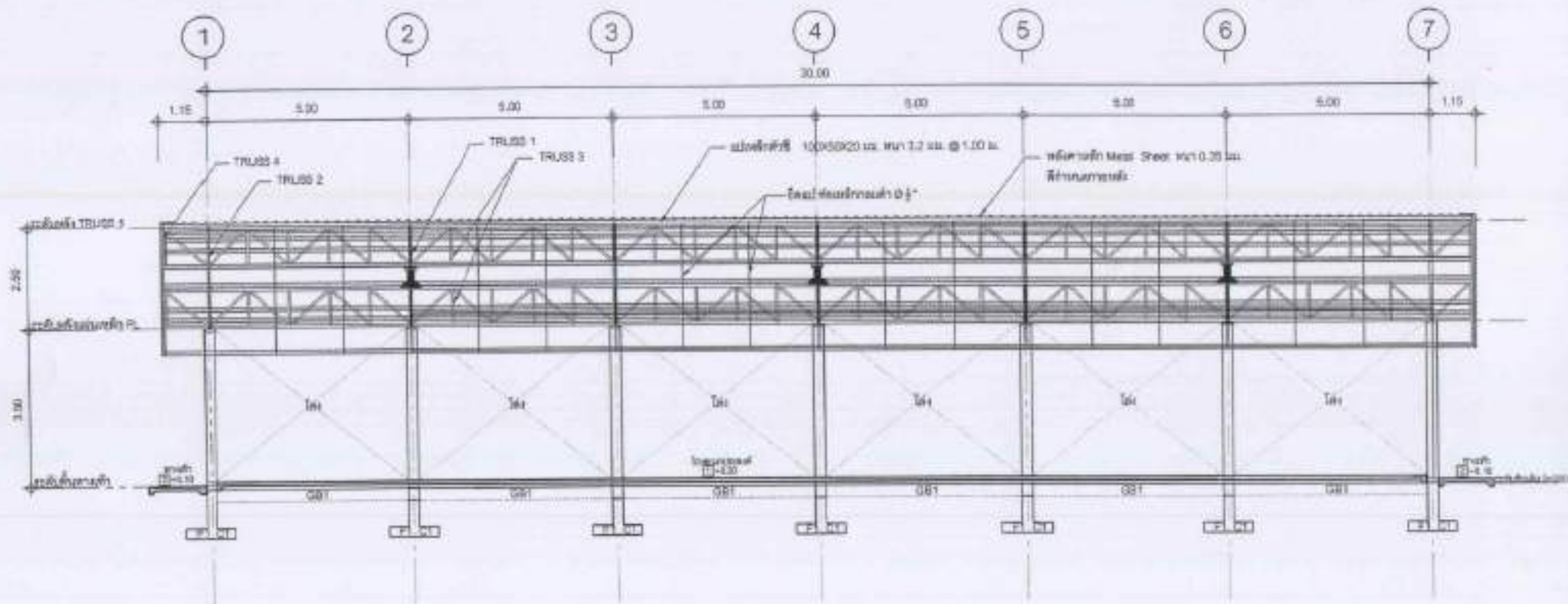
แบบแสดงรูปตัด B-B SCALE 1:100
