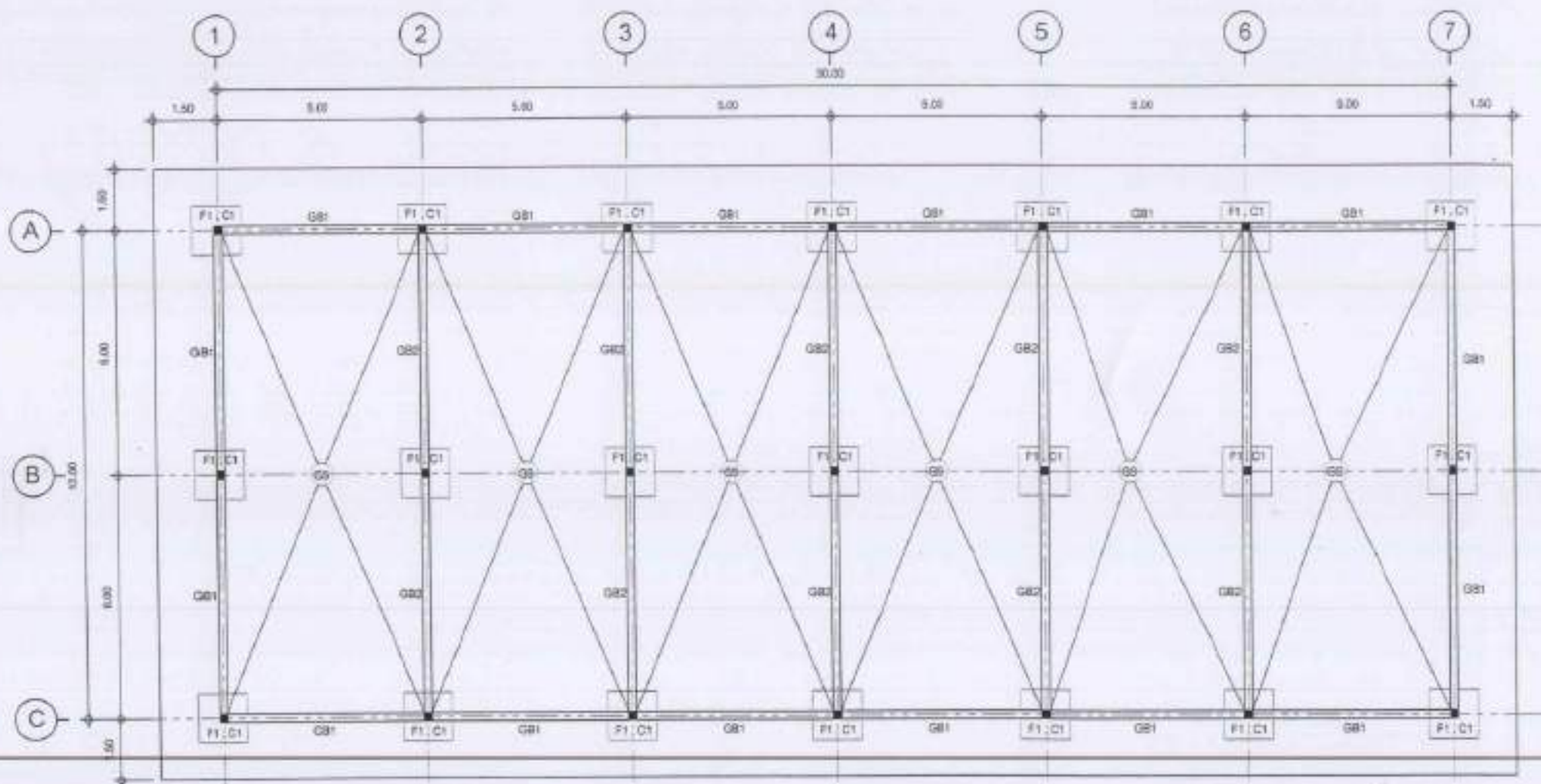
แบบแปลนฐานราก คาน เสาคาน SCALE 1/100
