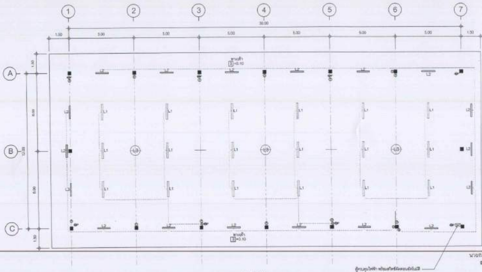
แบบแสดงแปลนไฟฟ้า
